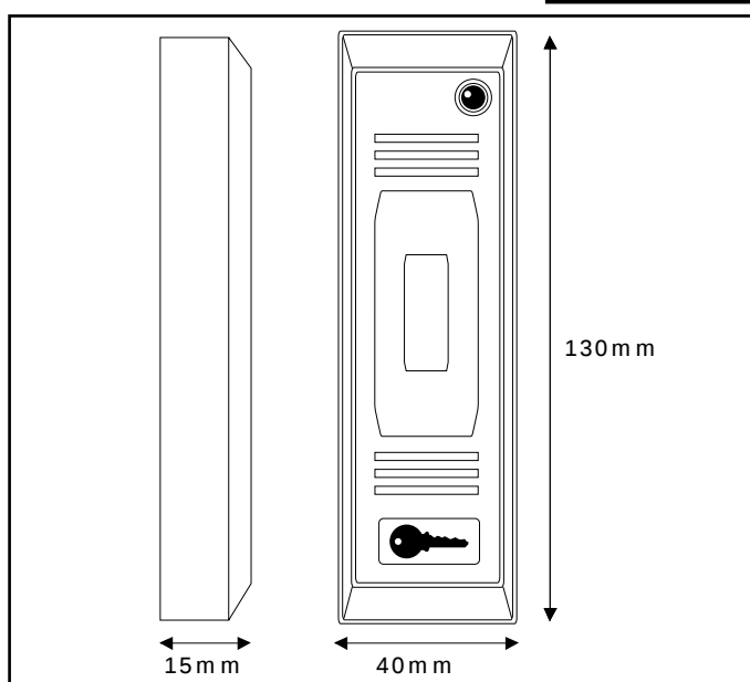
Dimensions
