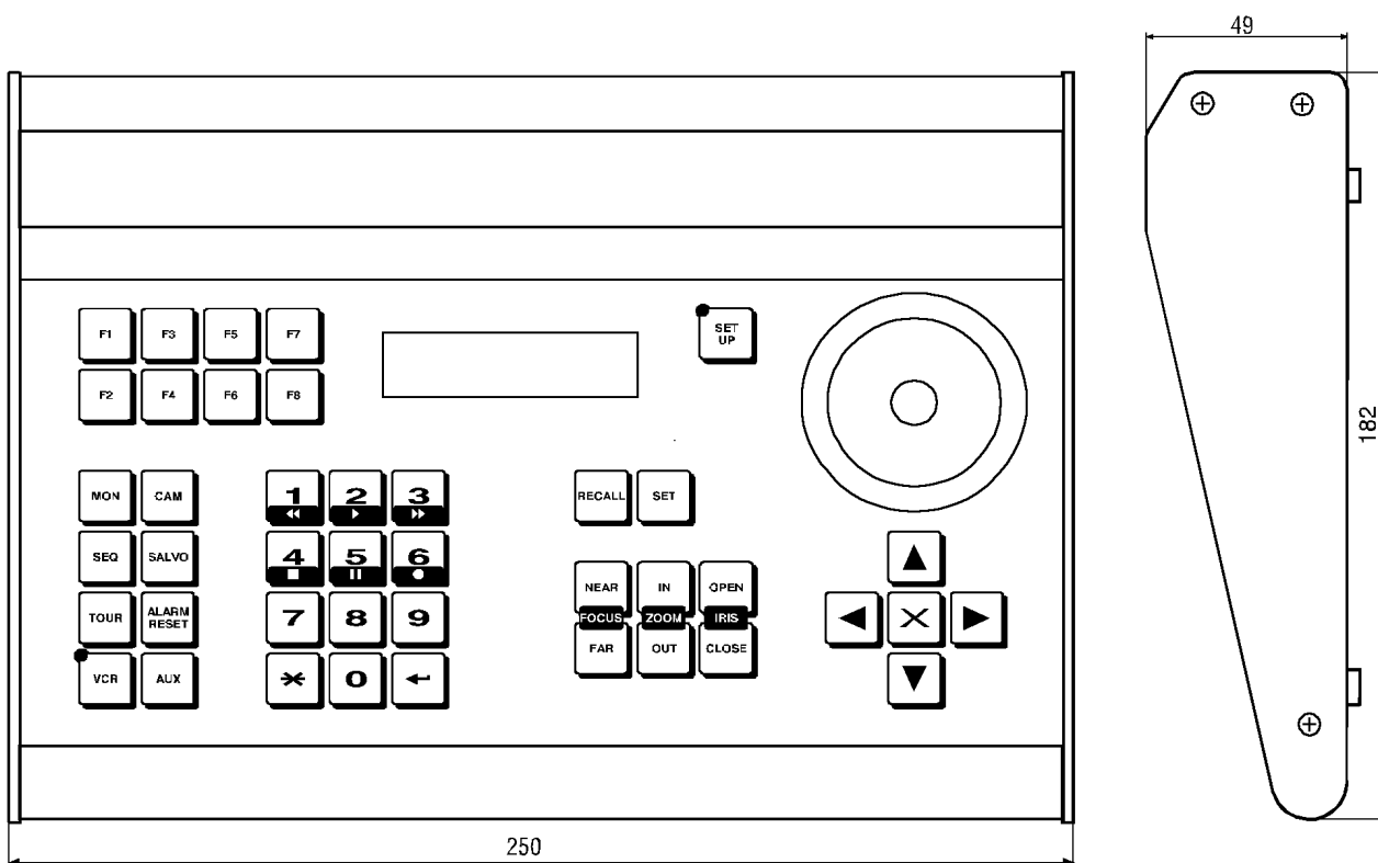
Maße/Dimensions: mm
