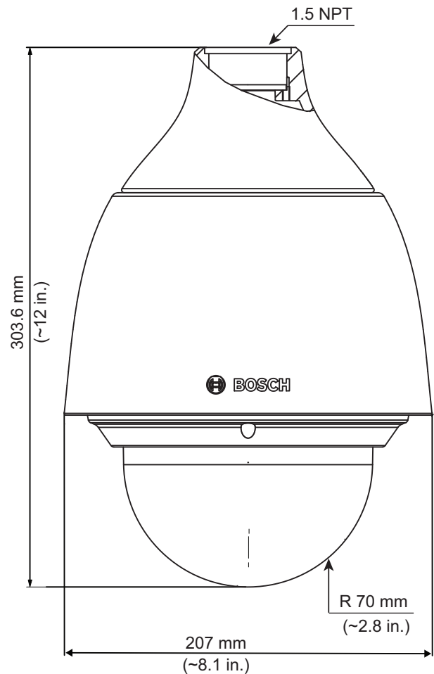
Fig. 7: Pendant model
